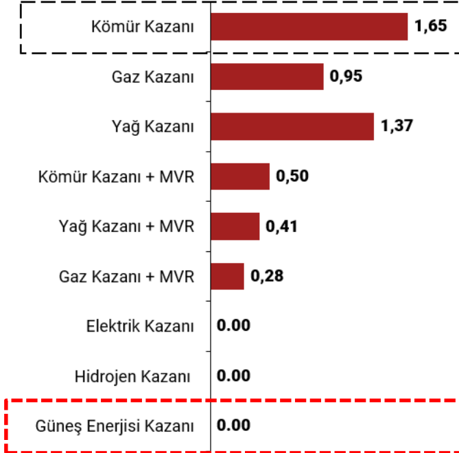
Kazan Teknolojilerinin Ortalama Emisyon Yoğunlukları (t CO2/t Al)
