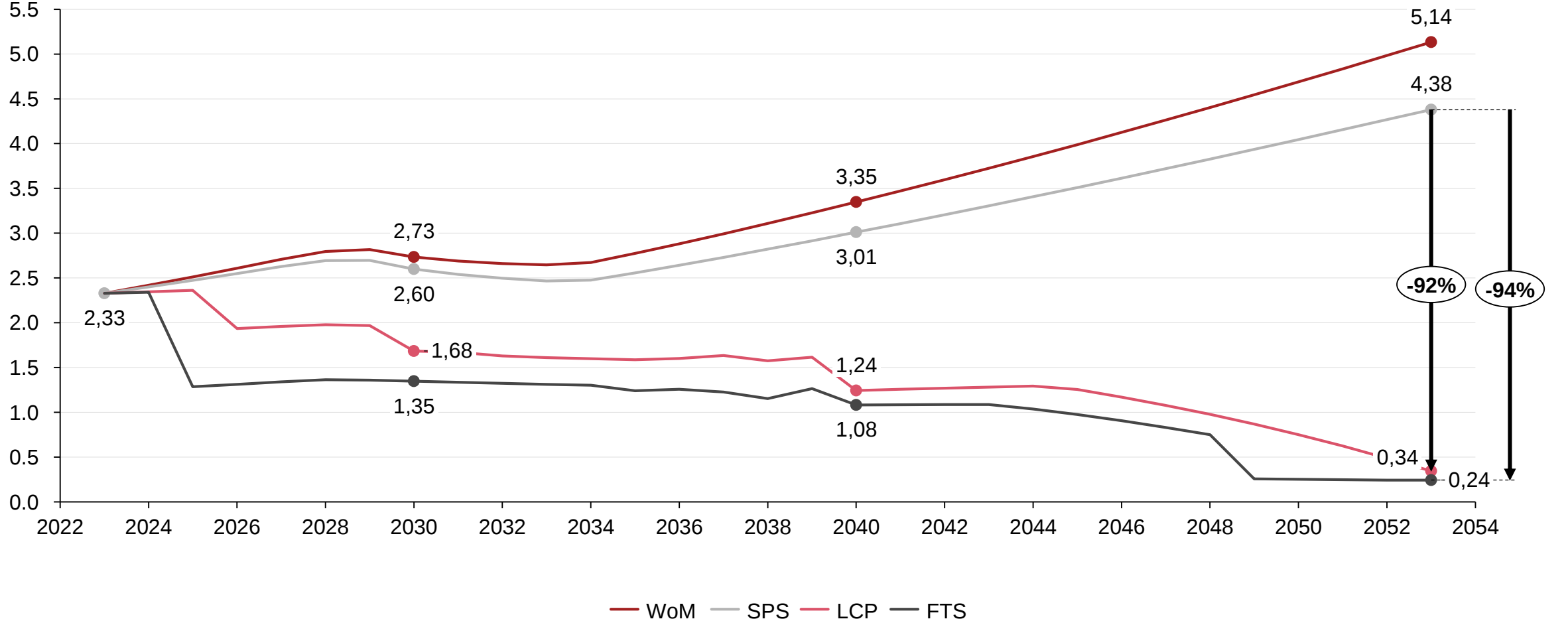
Toplam Emisyonlar (Milyon ton CO 2 e)
