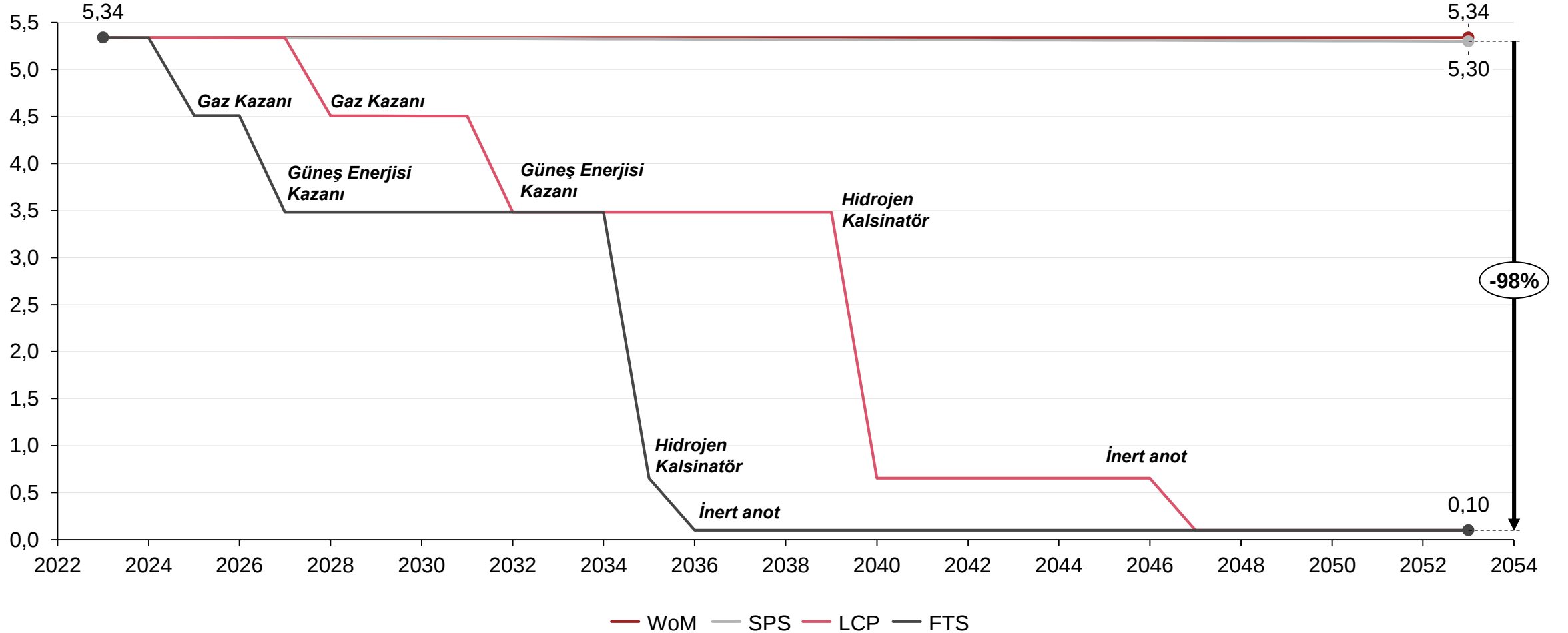
Emisyon Yoğunluğu (ton CO 2 e /ton Al)
