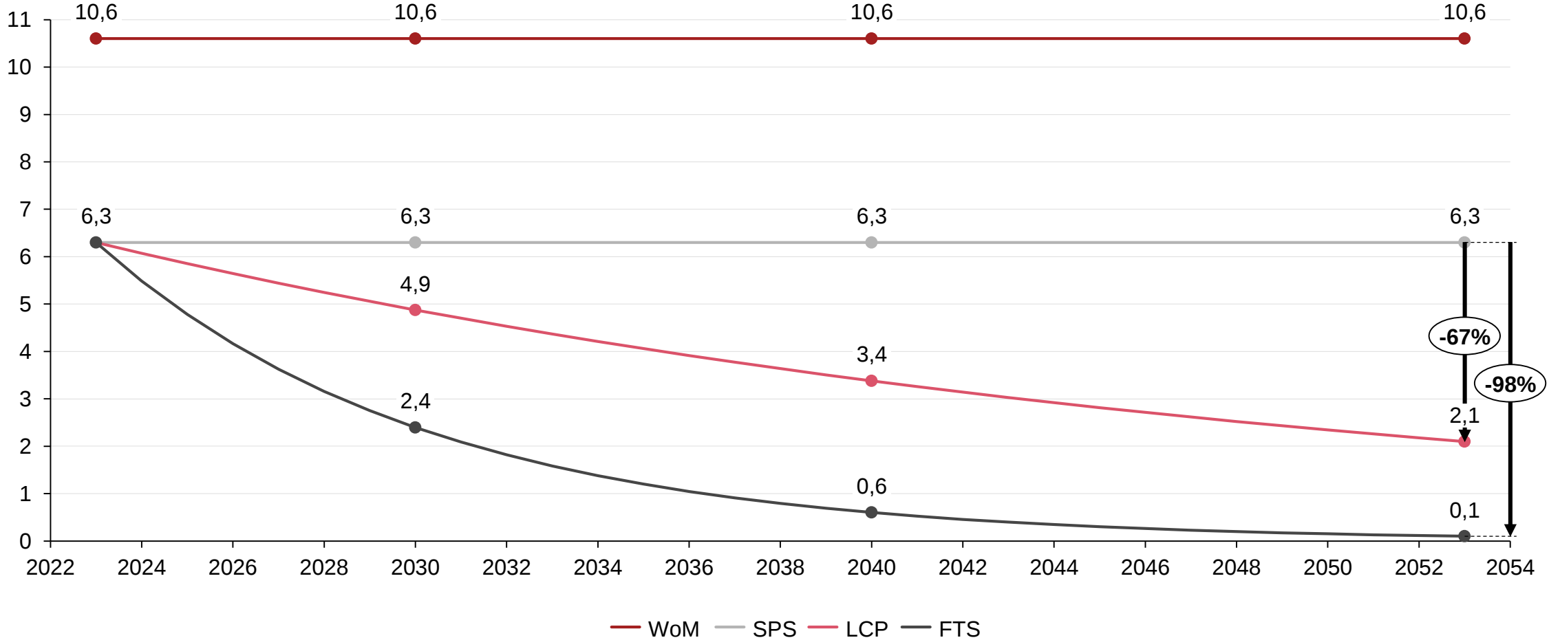
Emisyon Yoğunluğu (Girdi Kaynaklı Kapsam 3, ton CO 2 e / ton Al)
