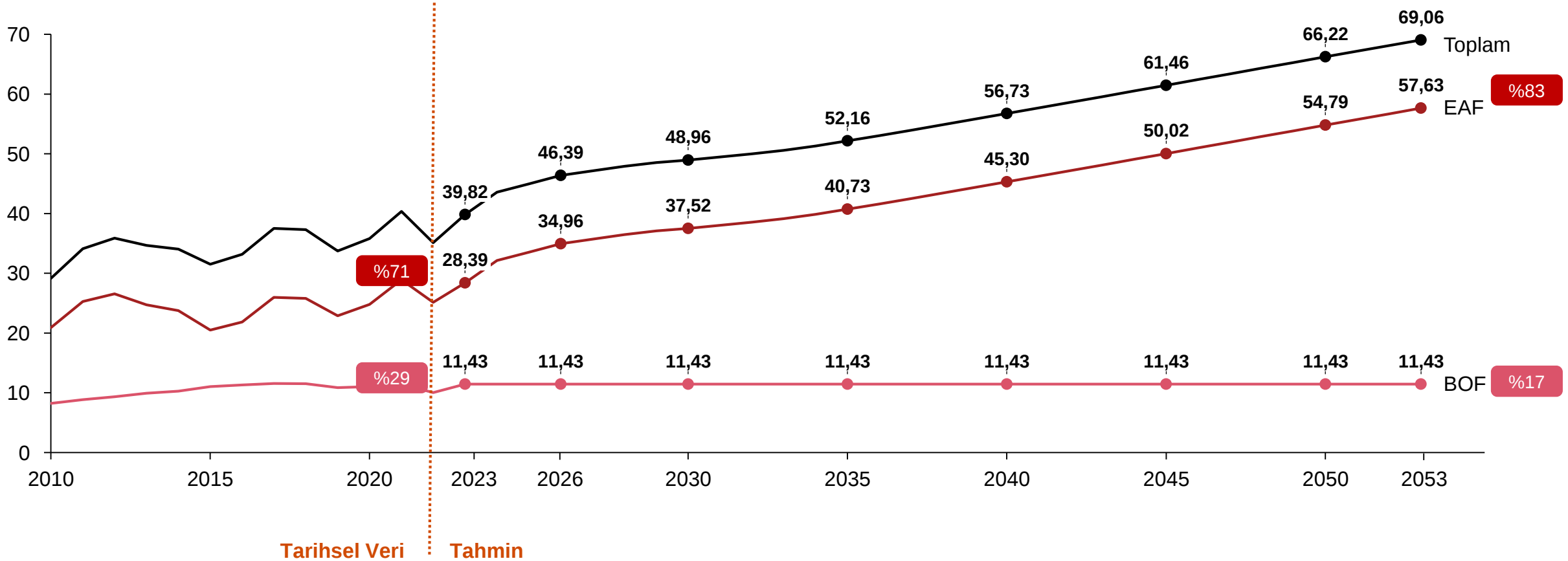
SPS Senaryosu için Çelik Üretim Yöntemlerine Göre Üretim Tahmini (Milyon Ton)
