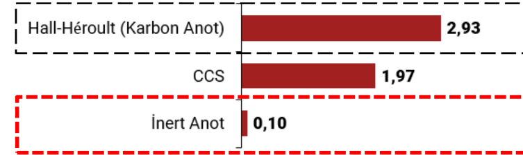
Anot Teknolojilerinin Ortalama Emisyon Yoğunlukları (t CO2/t Al)
